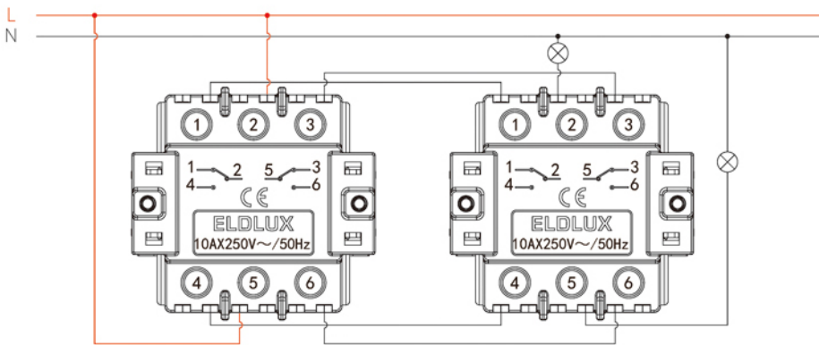
kettős váltókapcsoló (106 + 6)
