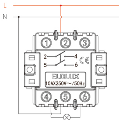
Kétpólusú kapcsoló (102)
