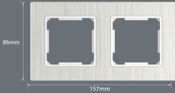
Kettes keret
