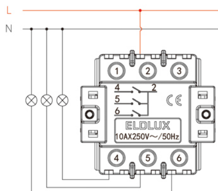
Hármas kapcsoló
