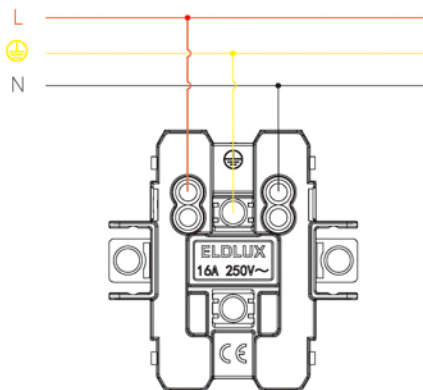
Dupla 2P+F csatlakozóaljzat
