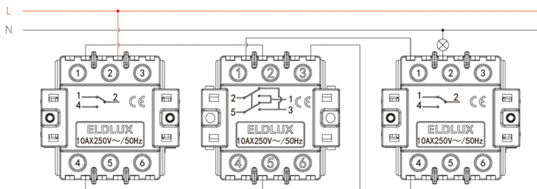
2 x Váltókapcsoló (106) + Kereszt váltókapcsoló (107)
