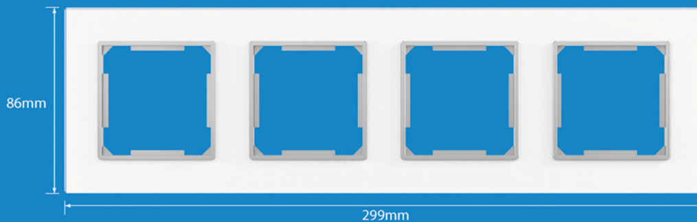
Négyes keret
