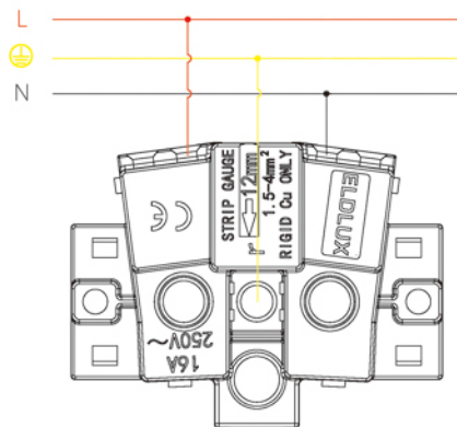
2P+F csatlakozóaljzat gyerekvédelemmel
