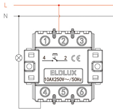
Nyomókapcsoló (101N)
