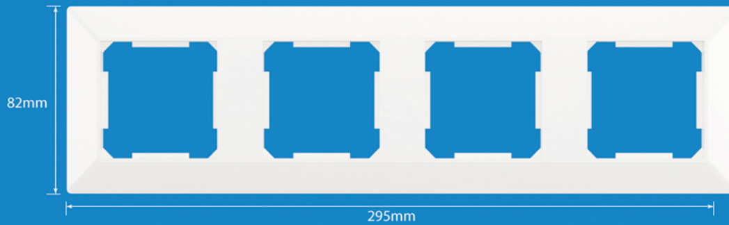
Négyes keret
