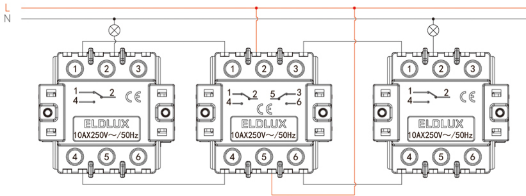
2 x Váltókapcsoló (106) + Kettős váltókapcsoló (106+6)
