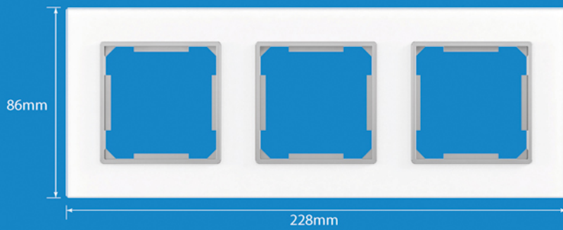
Hármas keret
