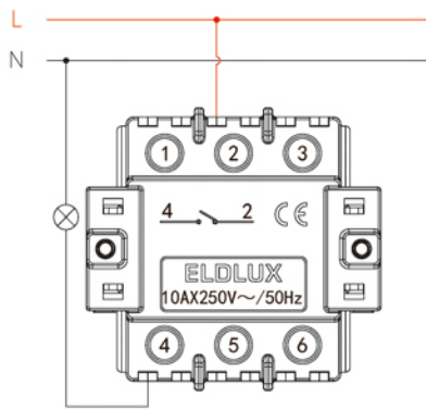
Egypólusú kapcsoló (101)
