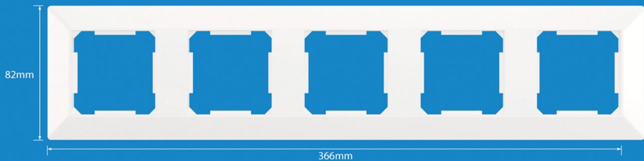
Ötös keret
